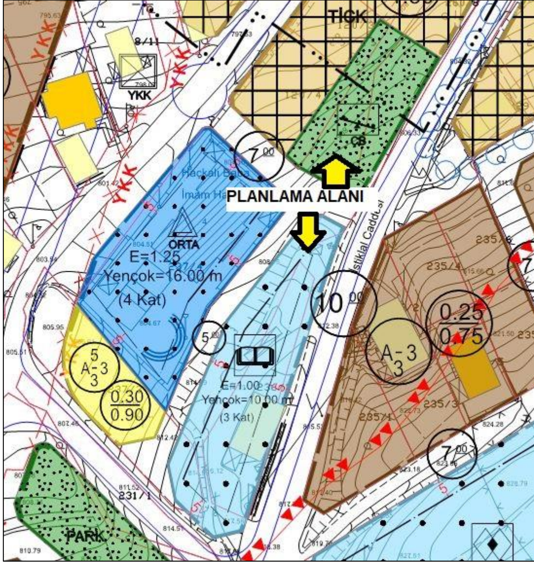
Şekil 10. Planlama Alanının 1/1000 ölçekli Uygulama İmar Planı
