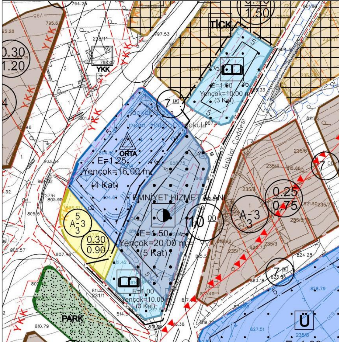
Şekil 12. Önerilen 1/1000 ölçekli Uygulama İmar Planı Değişikliği
